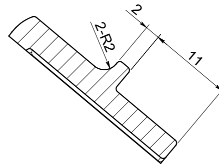
단면 A-A
