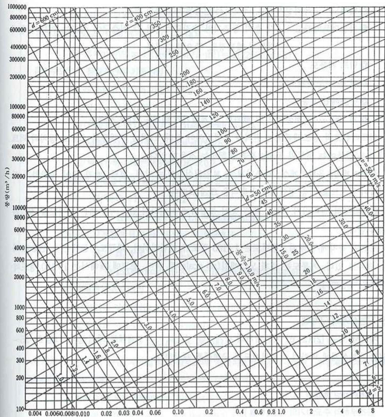
그림6-54, 덕트 摩擦抵抗線圖
