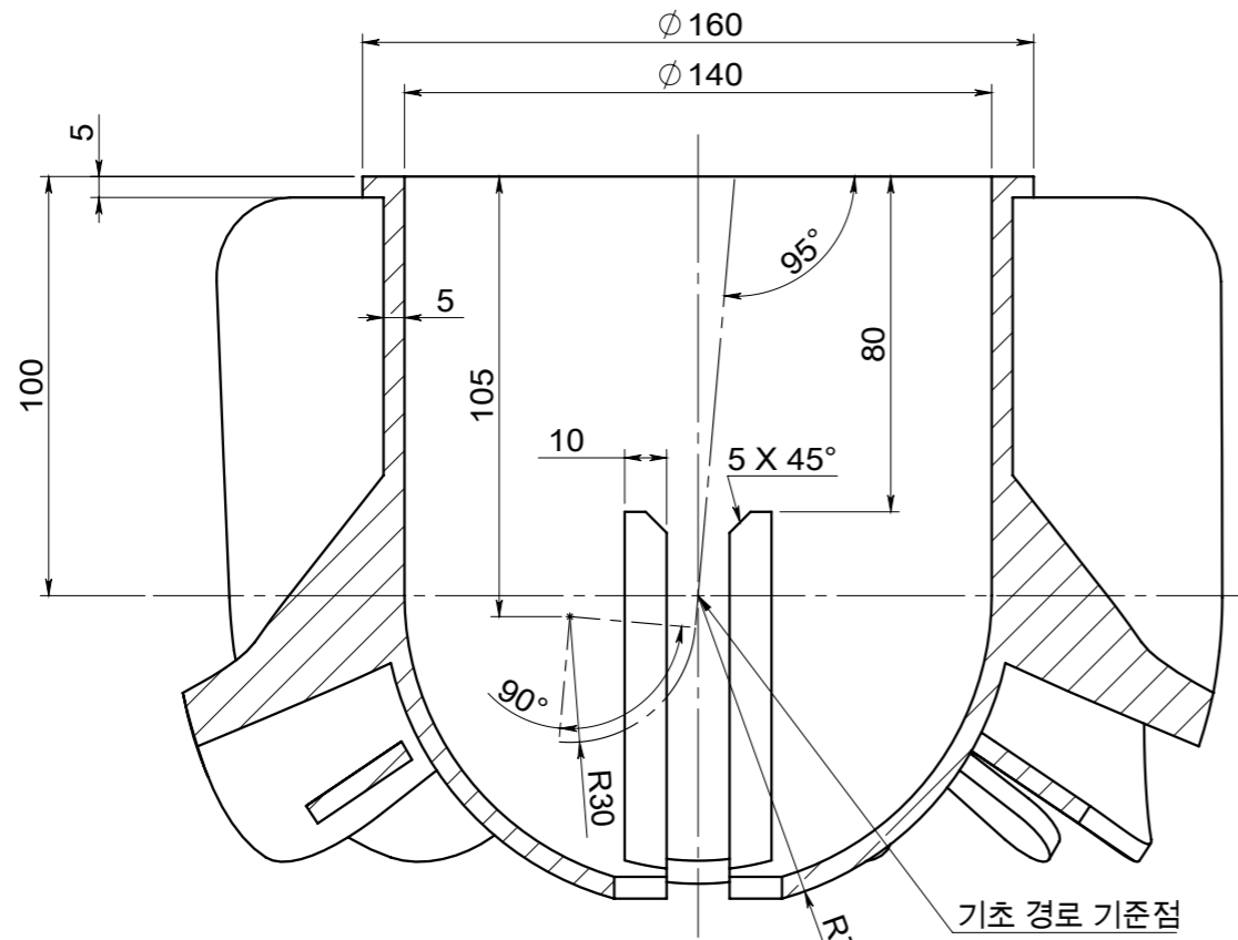
단면 A-A
