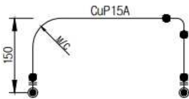
A - A' 단면도
