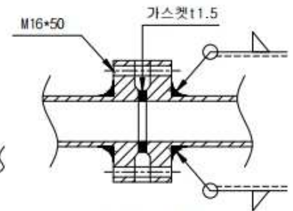
"C"부 상세도
