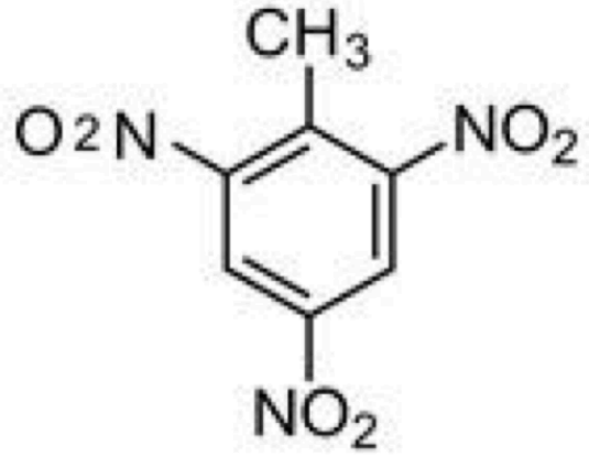
트리니트로톨루엔(TNT) 구조식
