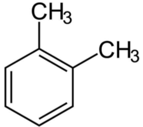
O-크실렌 구조식
