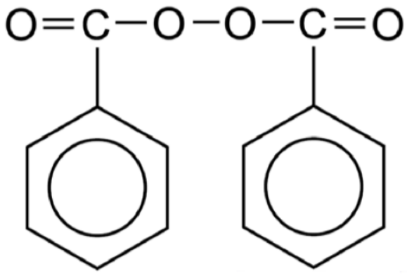
과산화벤조일
