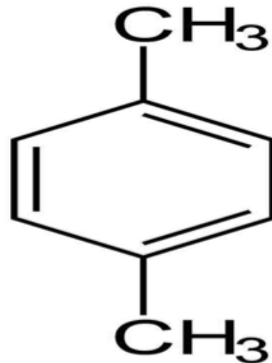
P-크실렌
