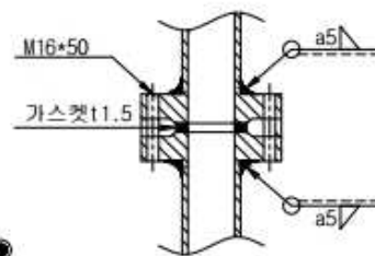
"C"부 상세도
