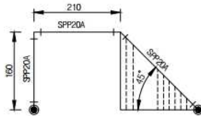
B - B' 단면도
