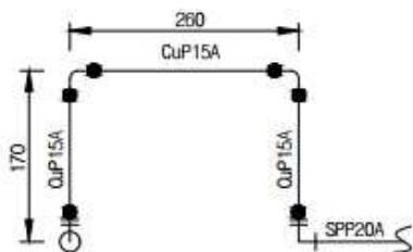
A - A' 단면도
