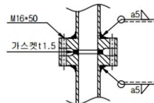
"B"부 상세도
