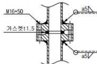
"B"부 상세도
