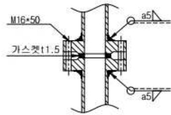
"B"부 상세도
