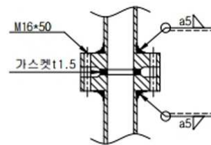
"B"부 상세도
