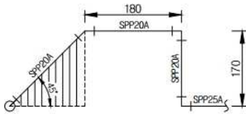
A - A' 단면도
