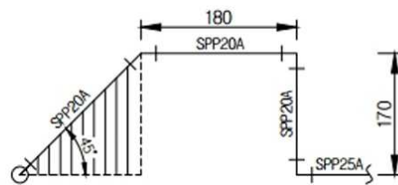
A - A' 단면도
