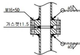
"B"부 상세도
