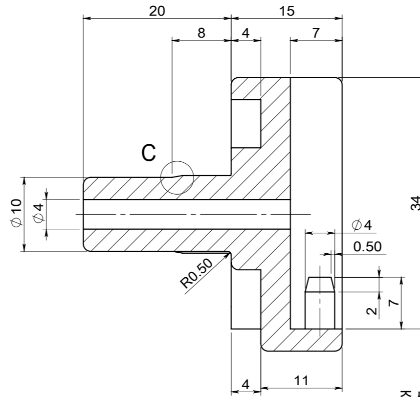
단면 A-A
