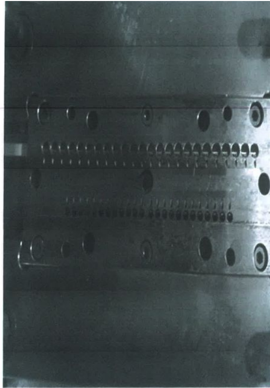
[ \Phi 4.5/\Phi 7 필터하우징 사출 금형 사진 2]
