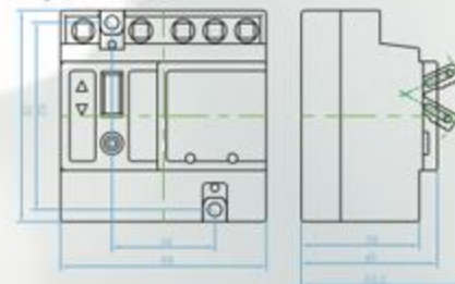
외형도/후부사이즈
