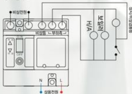
상세 결선도
