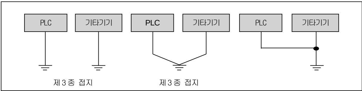
가) 전용접지: 가장 좋음 나) 공용접지: 양호 다) 공용접지: 불량
