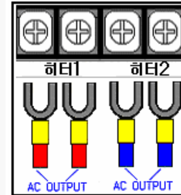
히터전원1, 히터전원2 결선
