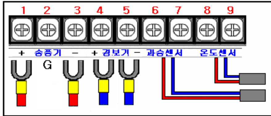
송풍기 및 센서결선
