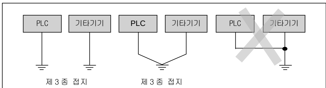
(a) 전용접지 : 가장 좋음
