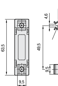
직렬형(S)
