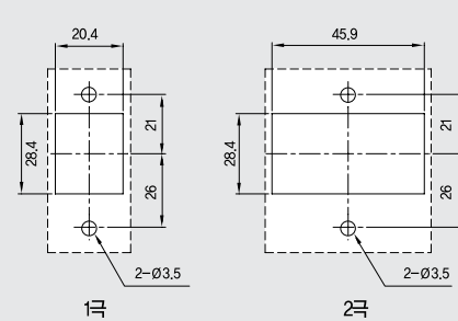
1극
