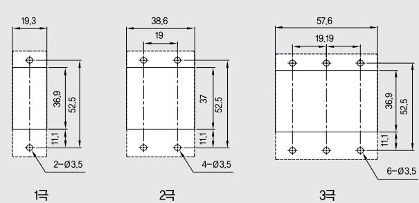
1극
