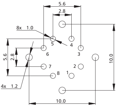
パネル取付寸法図
