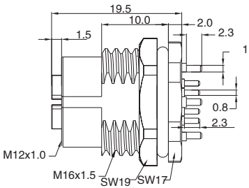
パネル取付寸法図
