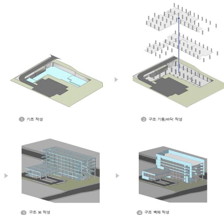
그림 12 구조 객체 작성 프로세스 예시
