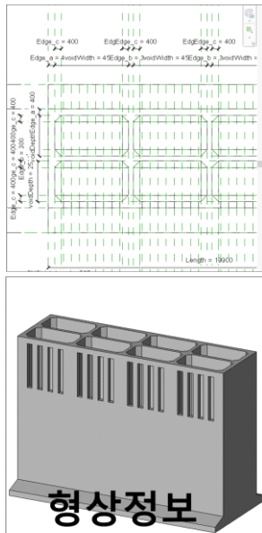
그림 24 BIM 라이브러리 작성 예시
