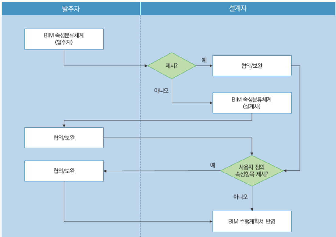
그림 21 BIM 모델 속성항목 협의 절차
