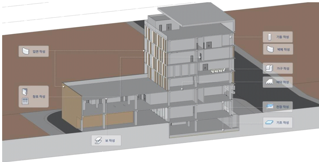
그림 7 계획설계 단계 부위 작성 대상 예시 [출처: 삼우종합건축사사무소, BIM 단계별 권장모델 참조, 2021]
